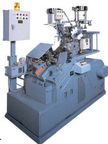
SRD120/10AV-3 センサーはオプションです
